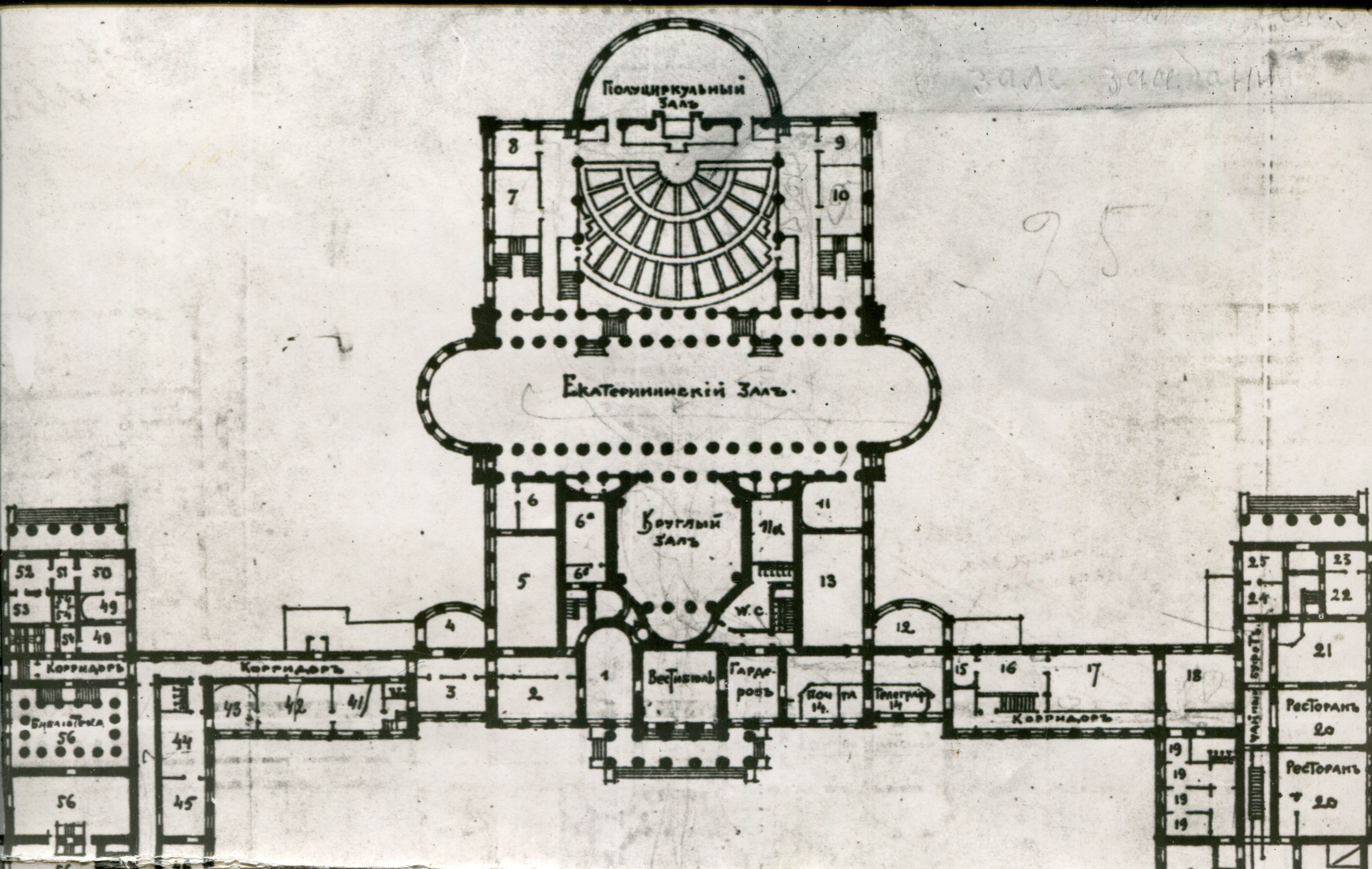
Планъ верхняго этажа.
